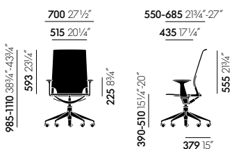
Meda Chair, mit Armlehnen
