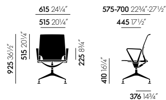
Meda Conference, mit polierten Aluminium-Ringarmlehnen
