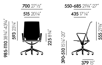
Meda Chair, mit polierten Aluminium-Ringarmlehnen
