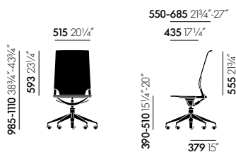
Meda Chair, ohne Armlehnen
