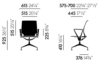
Meda Conference, mit Kunststoff-Ringarmlehnen
