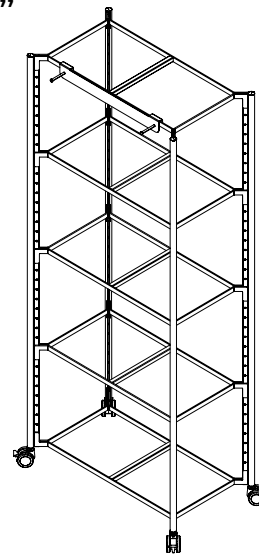
PIXEL RACK M 820x460,5x1935 mm mit PIXEL Whiteboard Halterung. with PIXEL whiteboard holder.
