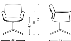
Drehstuhl mit 4-Fuß Swivel chair with 4-star base
