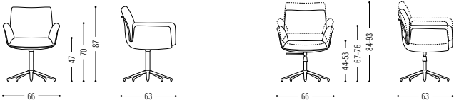
Drehstuhl mit 5-Fuß Gestell Swivel chair with 5-star base
