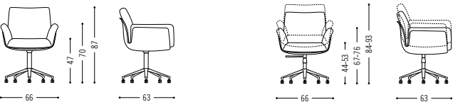
Drehstuhl mit 5-Fuß Gestell auf Rollen Swivel chair with 5-star base on castors
