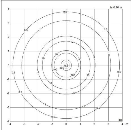
Isolux
