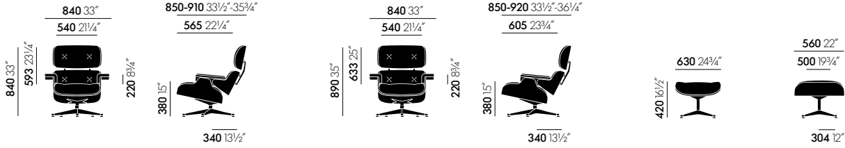
Lounge Chair, dimensions classiques
