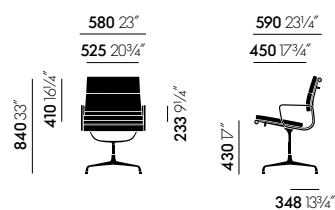
Soft Pad Chair EA 208 (hauteur classique), pivotant, avec accoudoirs
